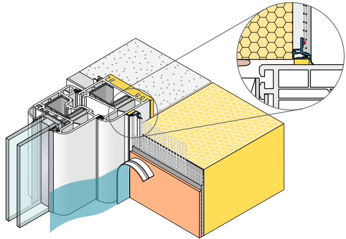
Anwendungszeichnung
