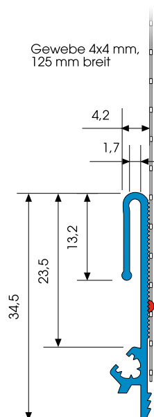
Schnittzeichnung in mm
